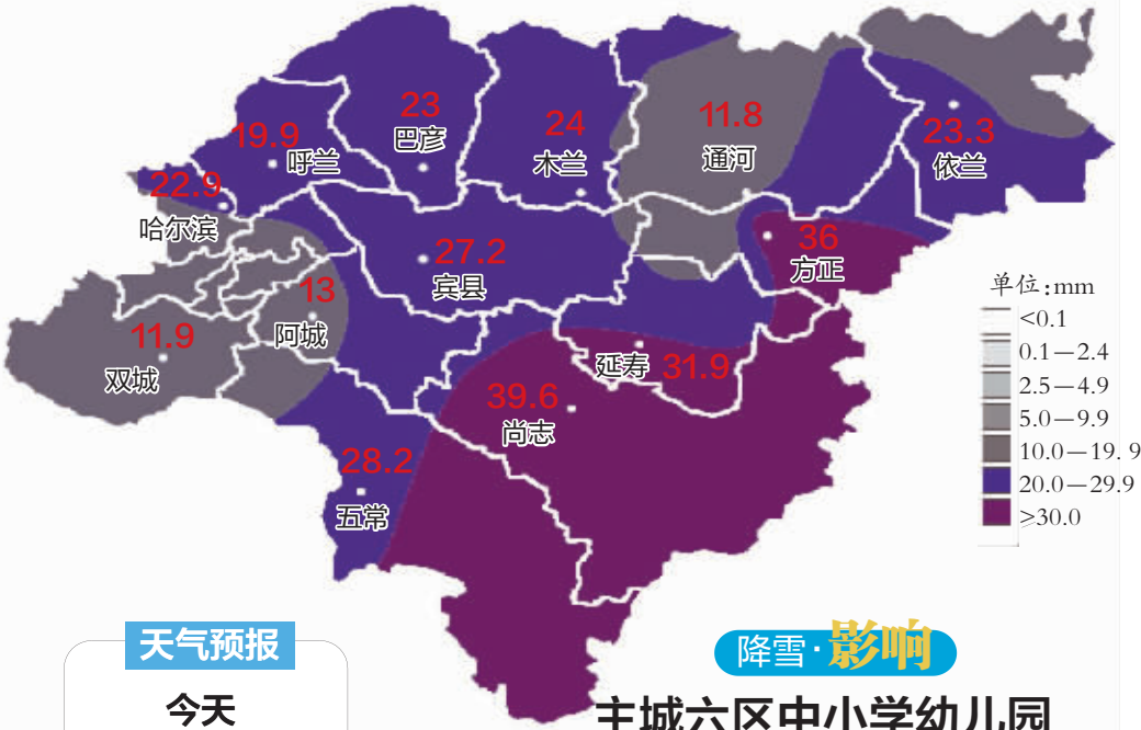
哈尔滨市降雪量分布图(单位:mm)
